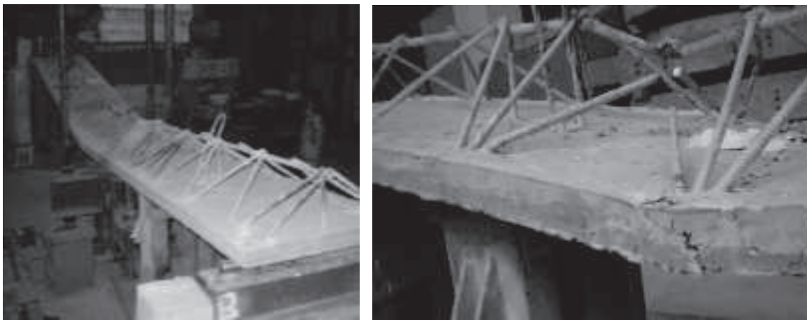
Рис.2 – Вигляд опалубкових залізобетонних плит після випробування:
