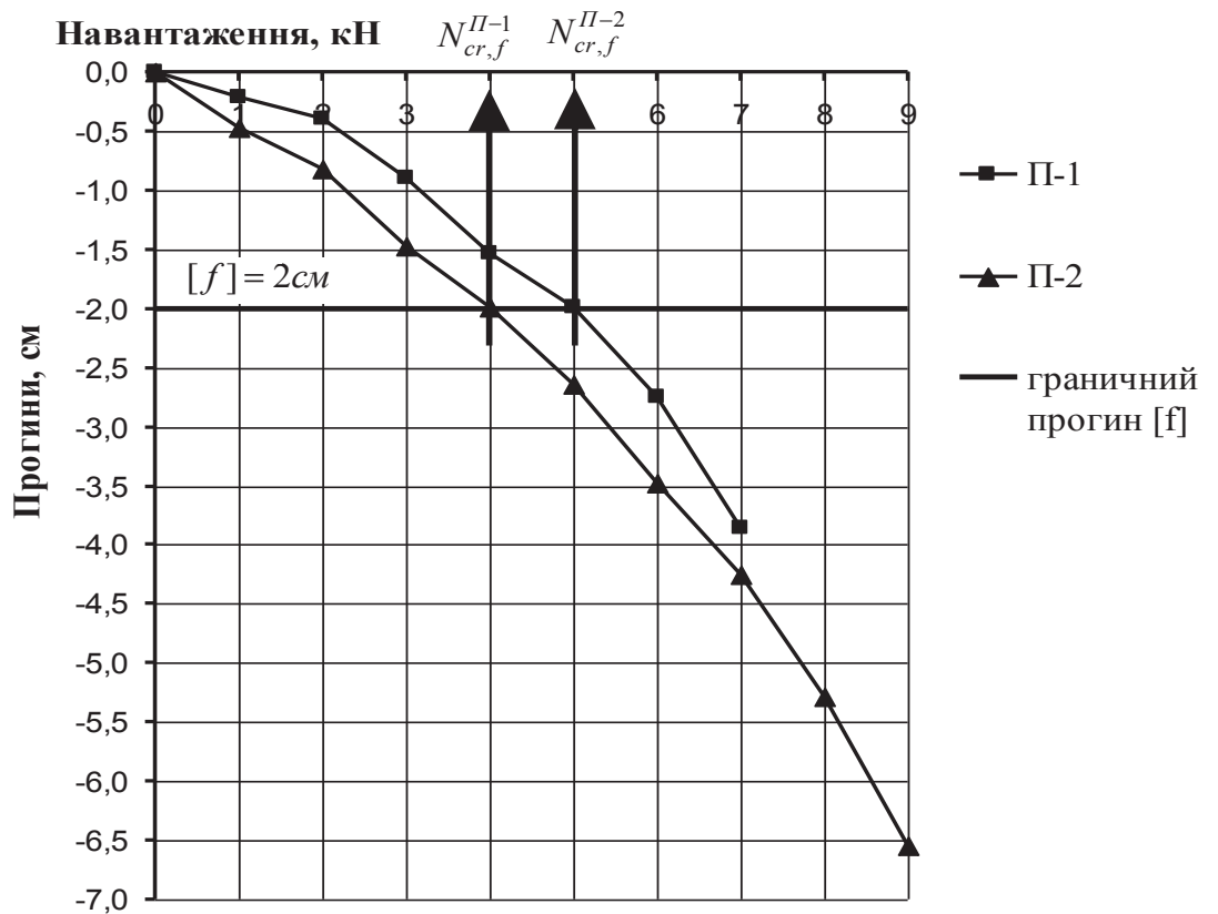
Рис.3 – Експериментальні залежності наростання прогинів опалубкових залізобетонних плит марок П-1 та П-2
